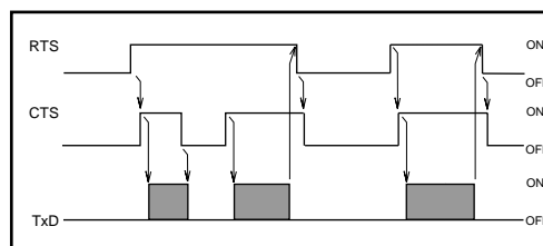
fig. 2.6; Modem protocol
